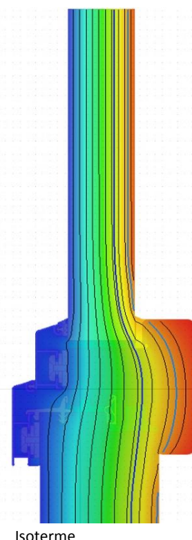
Isoterme
